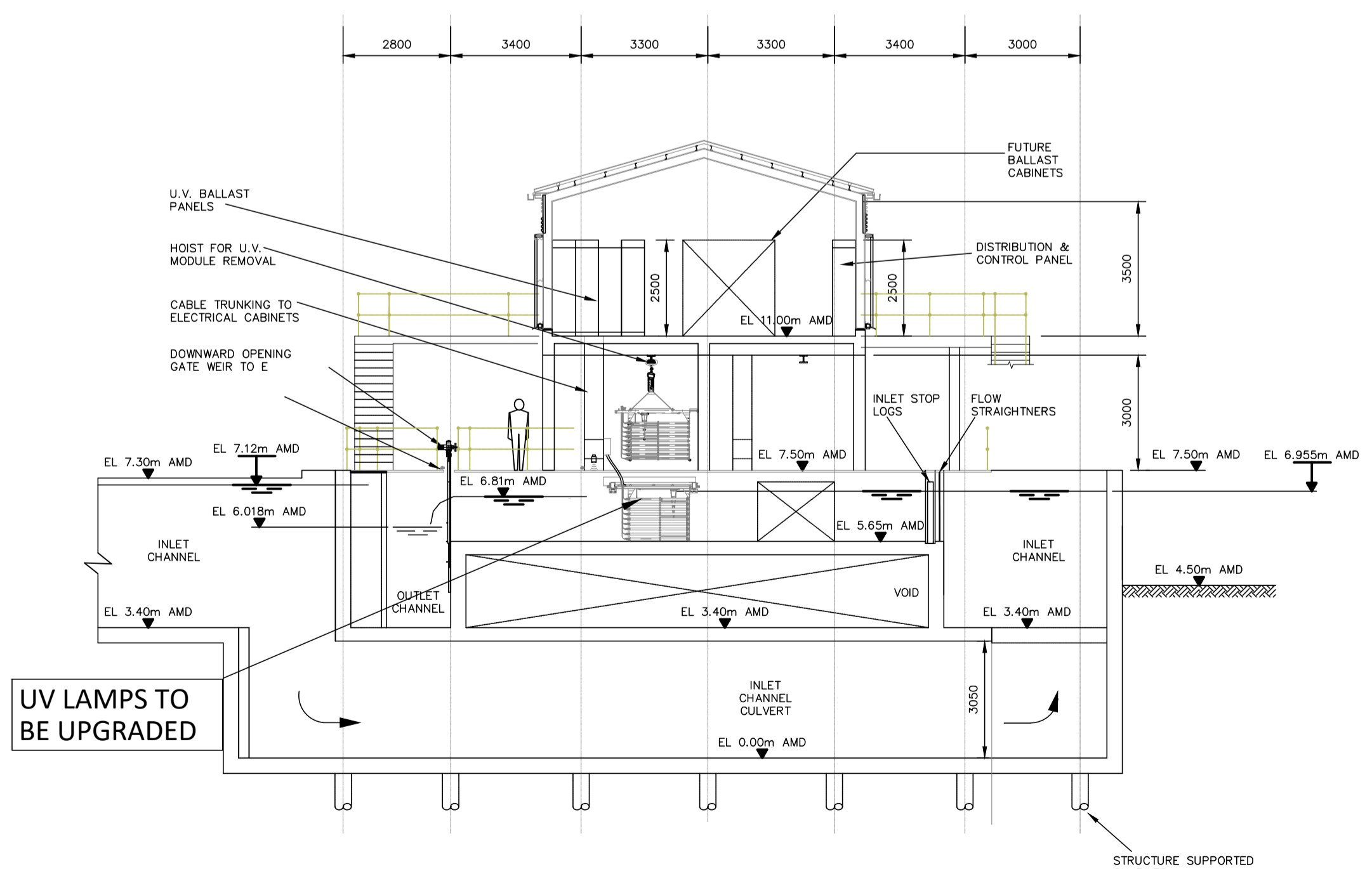
SECTION A-A
